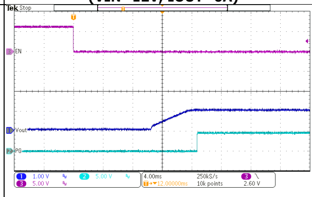
FIG.8 TURN-ON (VIN=12V, IOU=6A)
